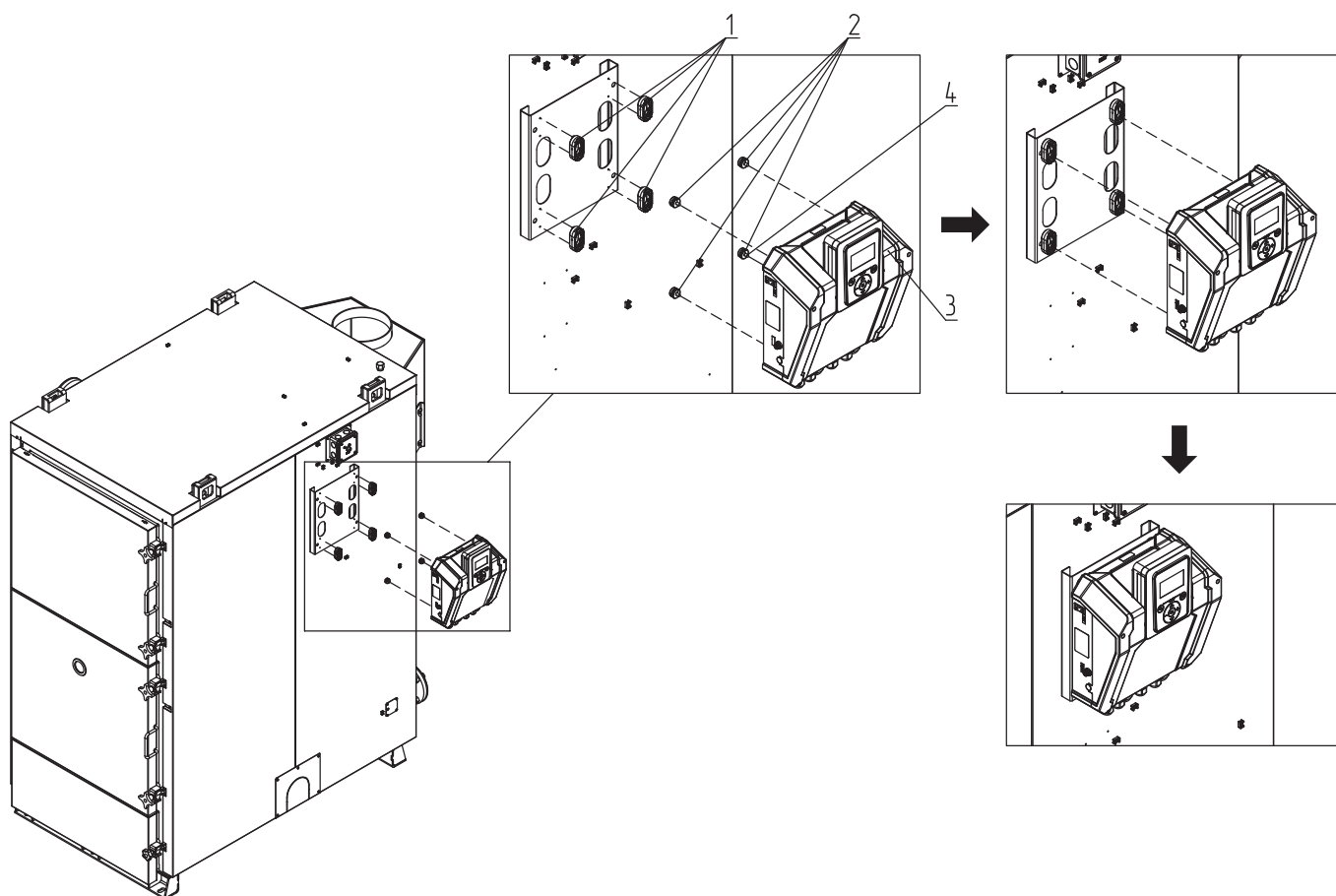
Рис.18 Монтаж контроллера
