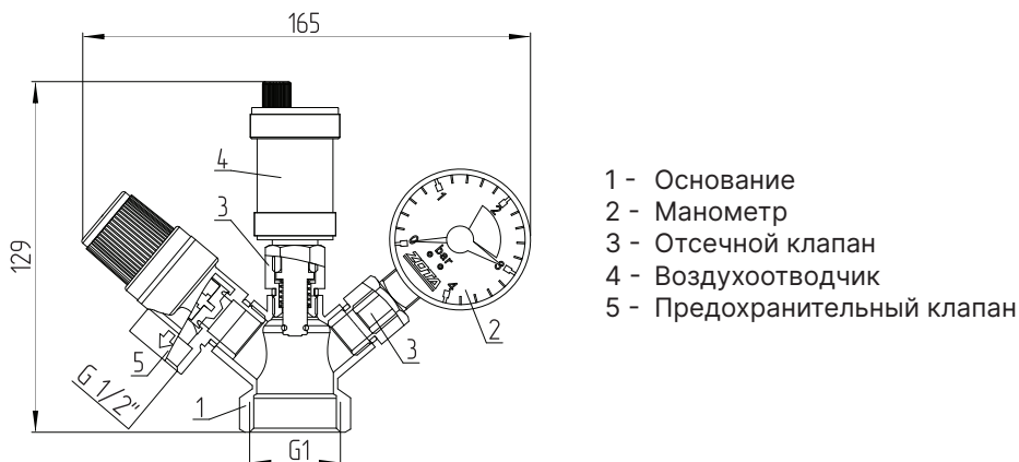
Рис. 3 Устройство группы безопасности котла 1" 3 bar ZOTA мини арт. GR4932007005
